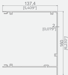
MOTOR KUTUSU PROFİLİ MOTOR BOX PROFILE
